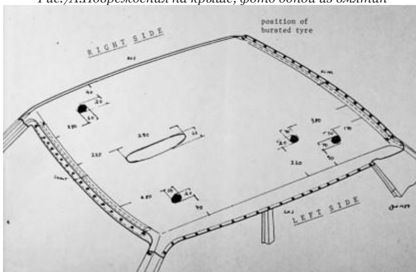
Рис.7Б. Повреждения на крыше, зарисовка
