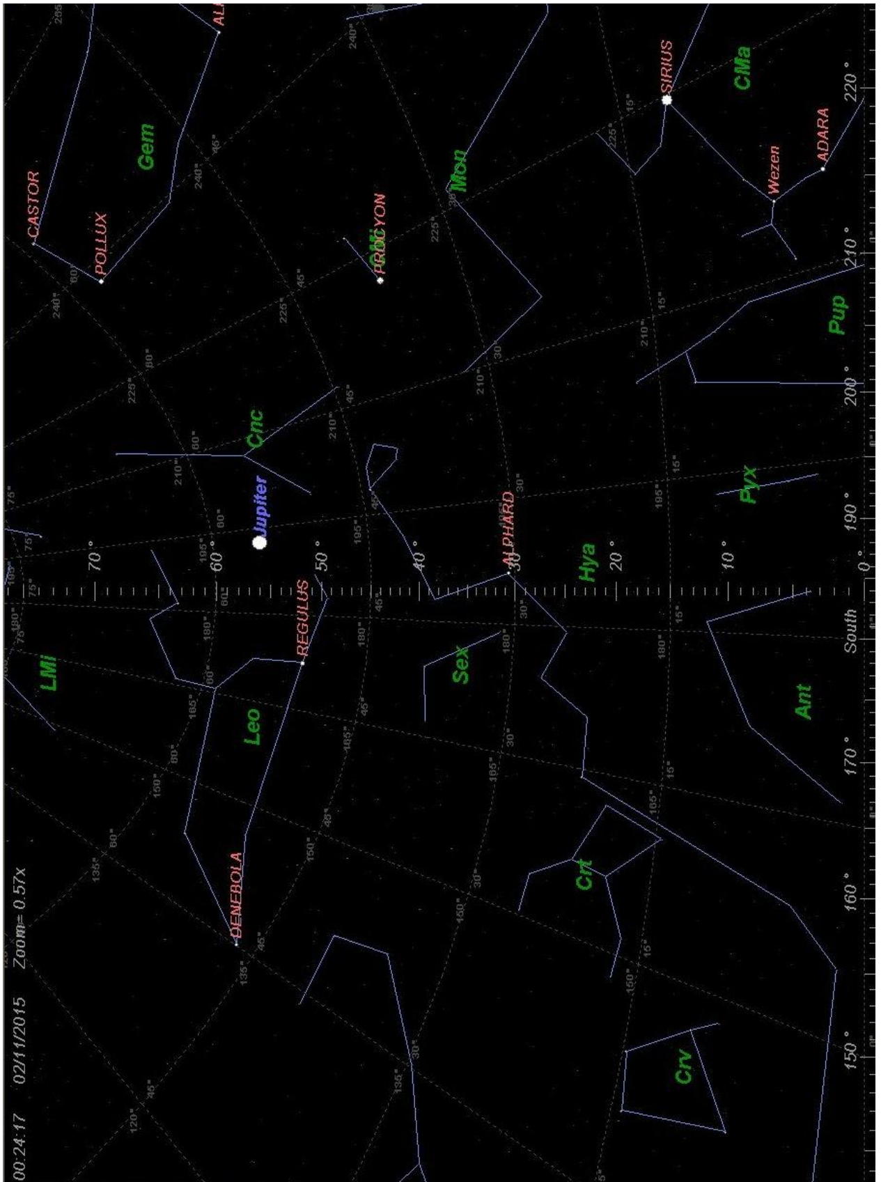
Рис.2. Місцезнаходження астрономічних об'єктів на небосхилі. Скріншот з програми WinStars.
