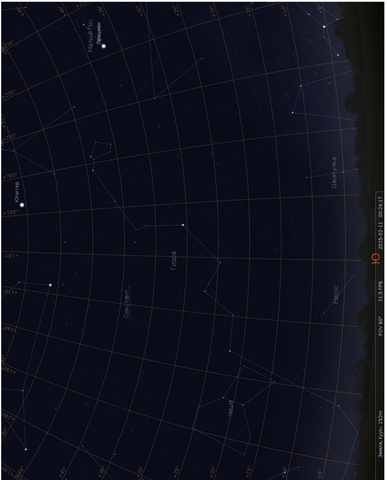
Рис.1. Місцезнаходження астрономічних об'єктів на небосхилі. Скріншот з програми Stellarium.
