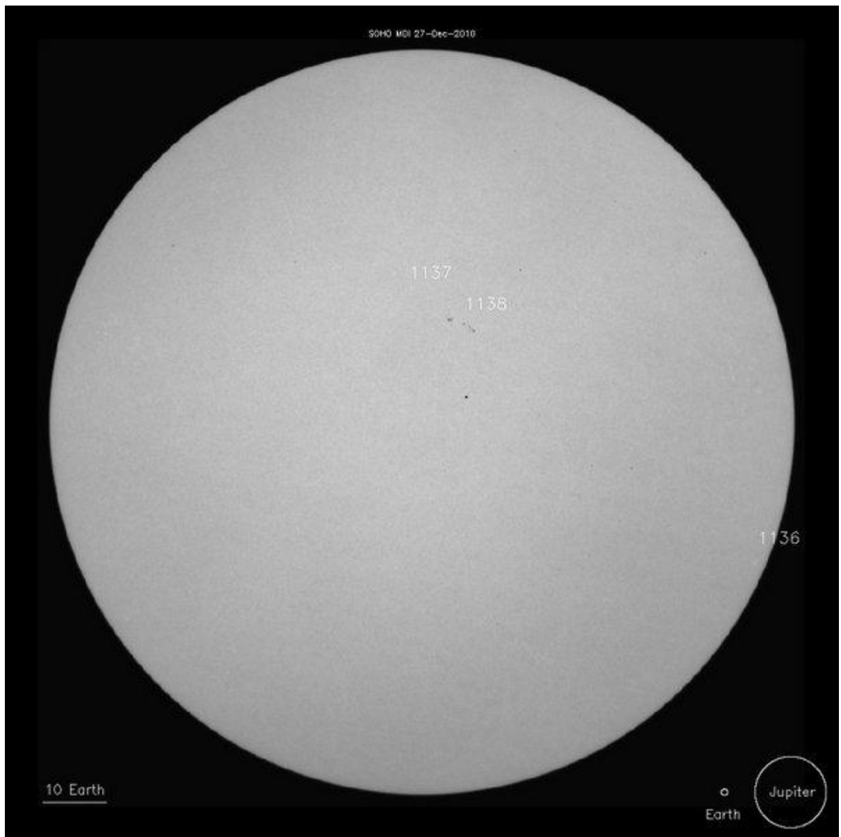
Два пятна на поверхности Солнца обнаружены с помощью аппарата SOHO 27 декабря 2010 года. NASA
