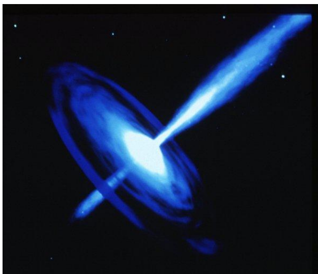
Так художники изобразили чёрную дыру в радиогалактике PKS 0521-36. Dana Berry (STScI)
