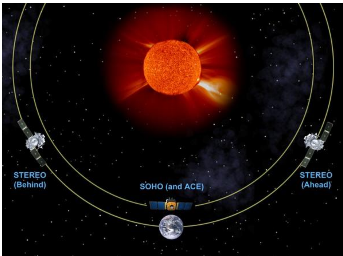
В начале 2011 года аппараты STEREO полностью облетят Солнце. NASA
