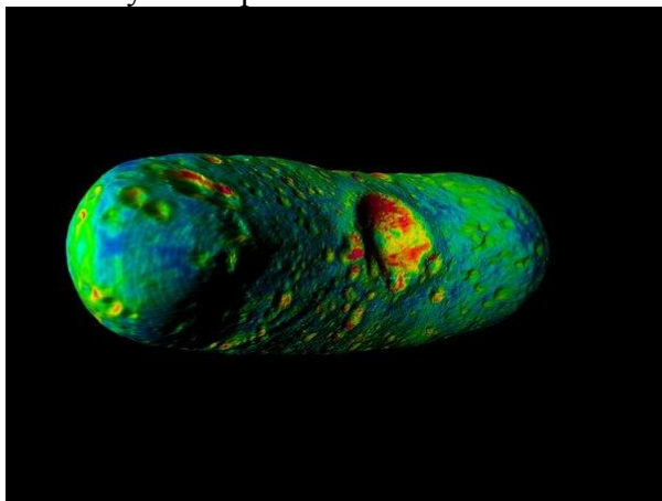
Астероид Эрос размером 433 метра пролетит 31 января 2012 года на расстоянии приблизительно 0,179 А.Е. Снимок космического зонда NEAR 14 февраля 2000 года. NASA Jet Propulsion Laboratory (NASA-JPL)
