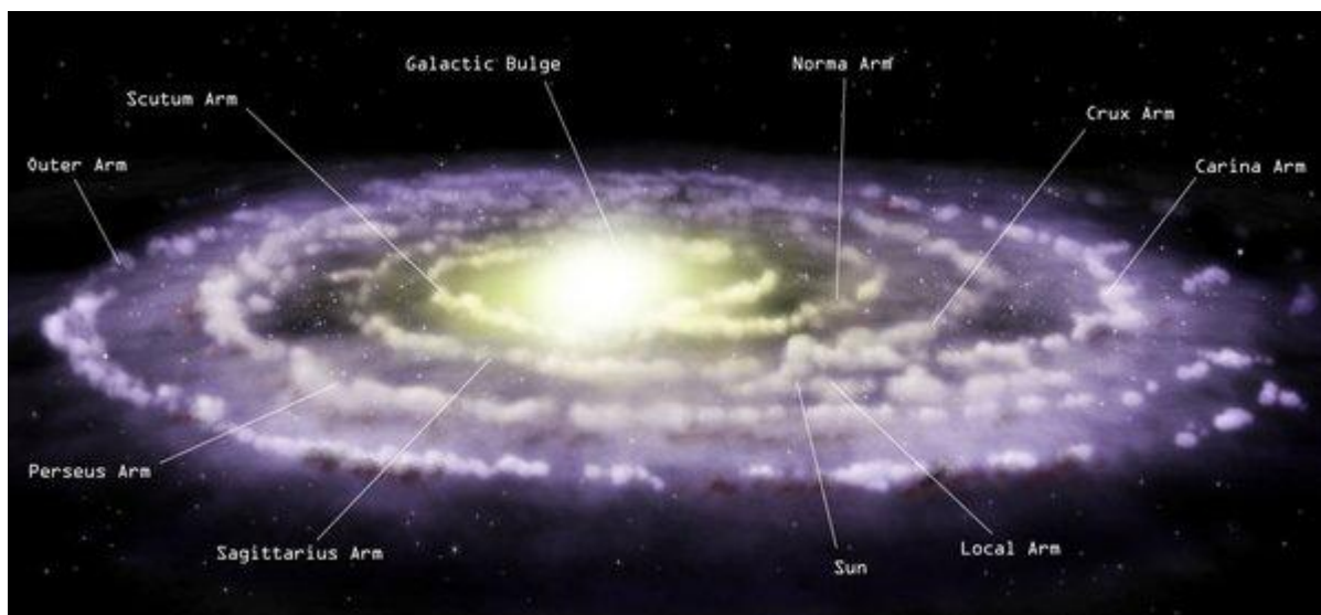
Галактика Млечный путь. NASA/CXC/M.Weiss
