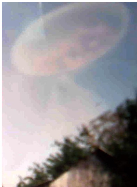
Рис. 2. Летинкулярное облако
