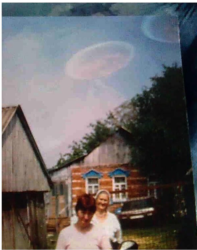
Рис.1. Летинкулярные облака
