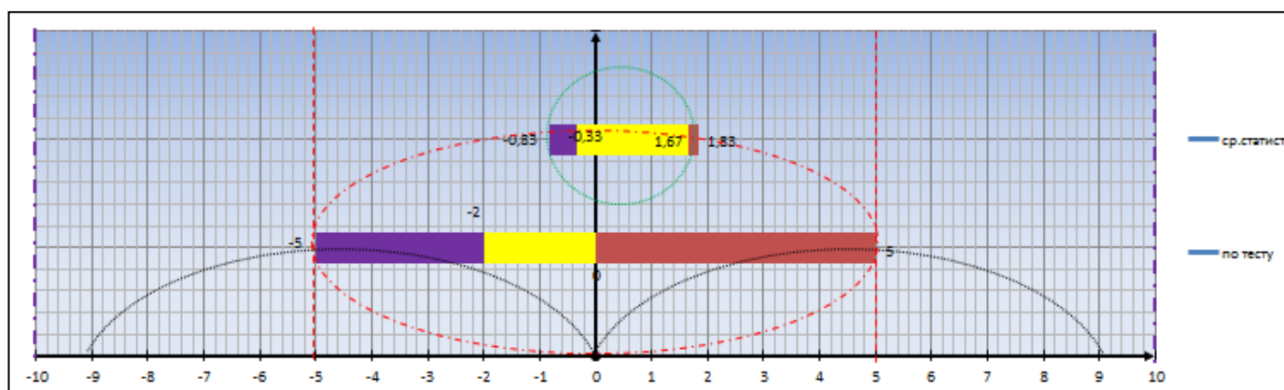
ДИАГРАММА СООТНОШЕНИЙ СИСТЕМНОГО И ВНЕСИСТЕМНОГО В ДИНАМИКЕ НЕСОЗНАТЕЛЬНОГО
