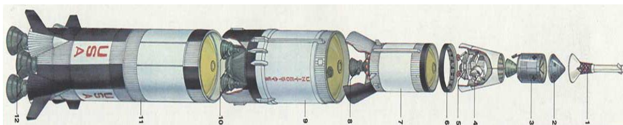
Рис.1.Ступени ракеты «Сатурн-5».
