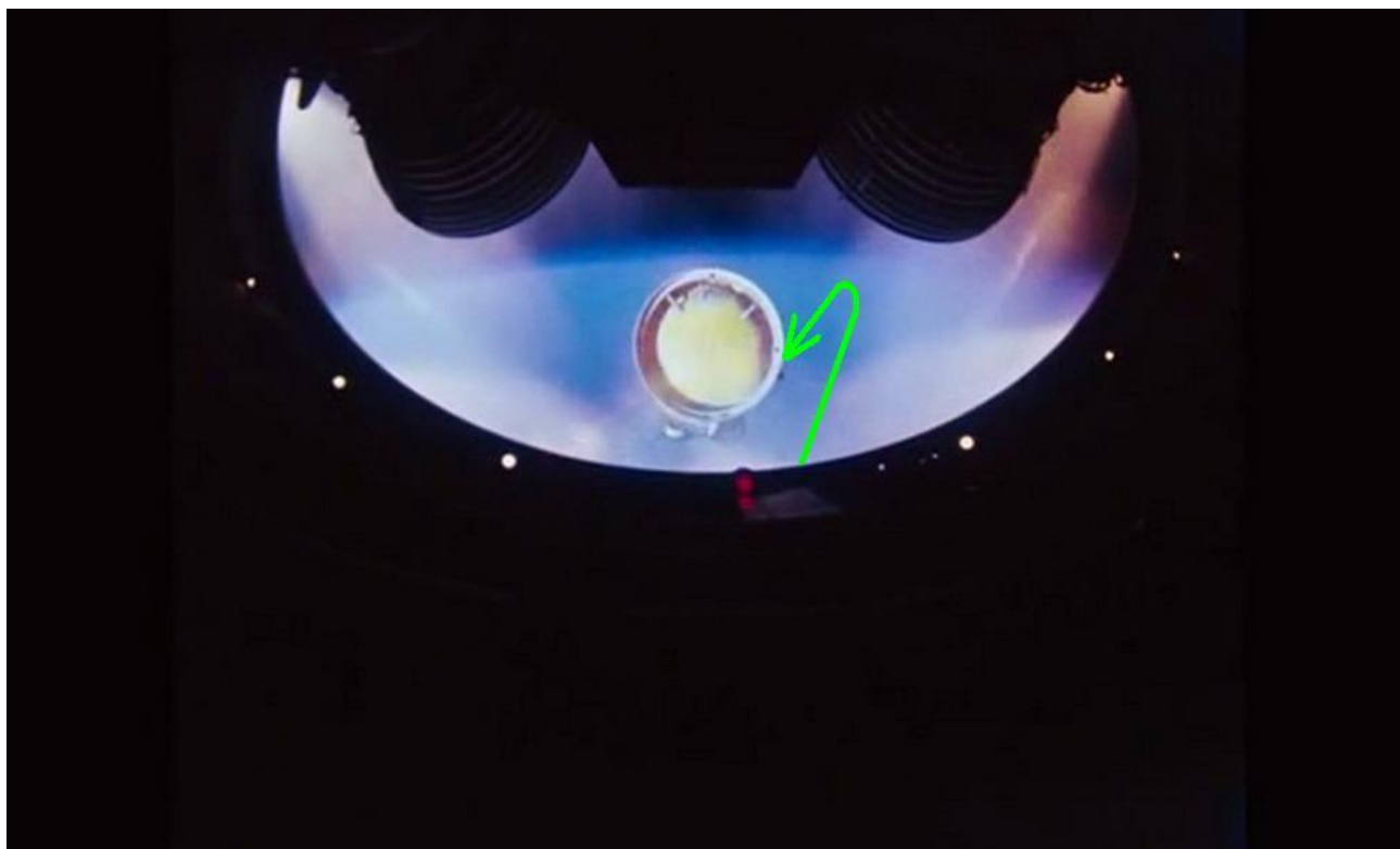
Рис.25.Траектория пролёта нло при расстыковке ступени ракеты «Сатурн-5» миссии «Аполлон-11».
