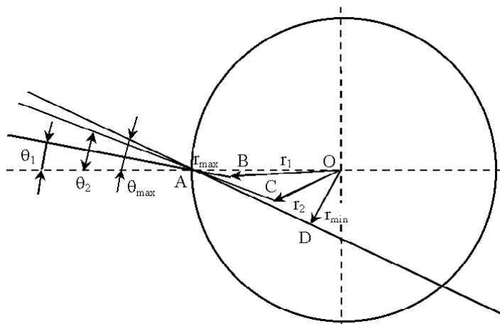
Рис. 1. Геометрия, отражающая результаты измерения границы зоны. O – центр зоны, A, B, C, D – точки встречи и соответствующие им радиусы r_{\max} , r_1 , r_2 и r_{\min} . 0 < \theta_1 < \theta_2 < \theta_{\max} , r_{\max} > r_1 > r_2 > r_{\min} .
