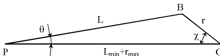
Рис.3. Схема для определения взаимосвязи параметров угловых гониметров.
