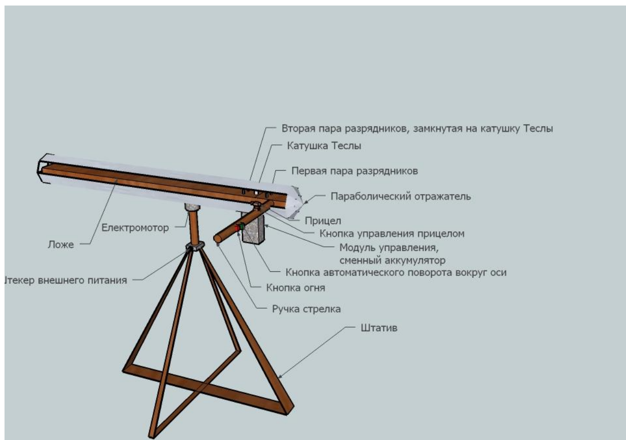
Рис.3. СШП-генератор (Миронов Н., УНИЦА)
