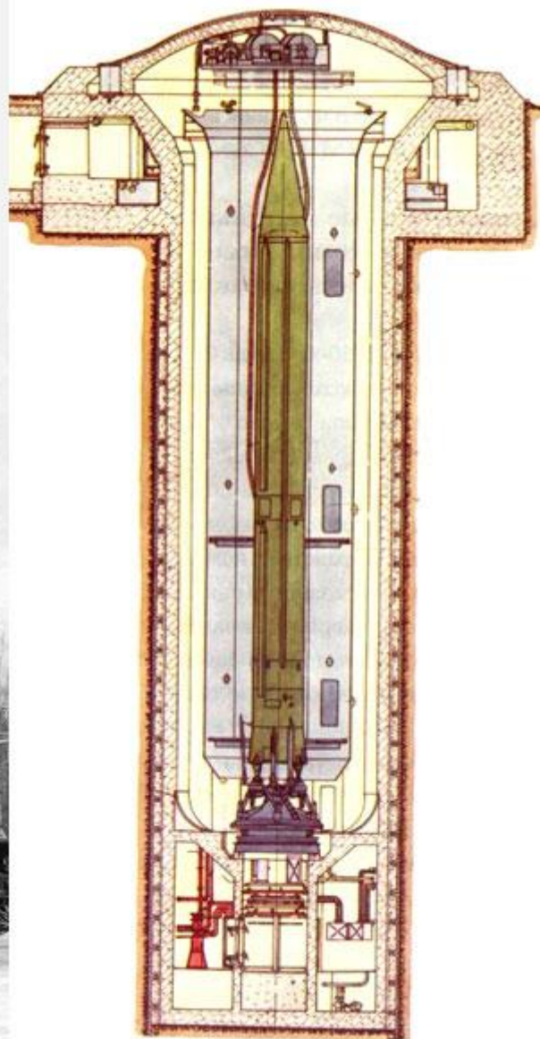
Ракета Р-12: подготовка к наземному старту (слева) и шахтный вариант (справа).
