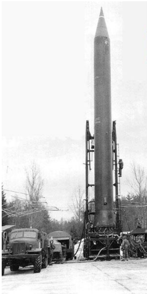
Ракета Р-12: подготовка к наземному старту (слева) и шахтный вариант (справа).
