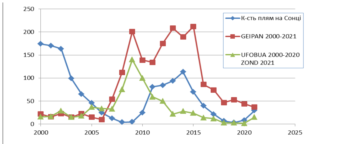
Рис.12. Кореляції сонячної активності (числа Вольфа) та кількості повідомлень у первинних масивах
