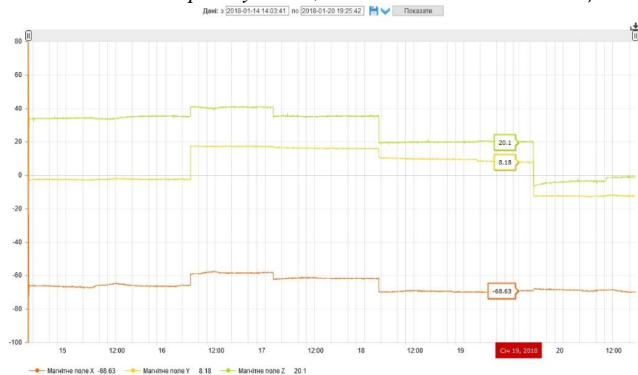
Рис.8. Аномальні сплески магнітного поля між 16 та 19 січня 2018р.
