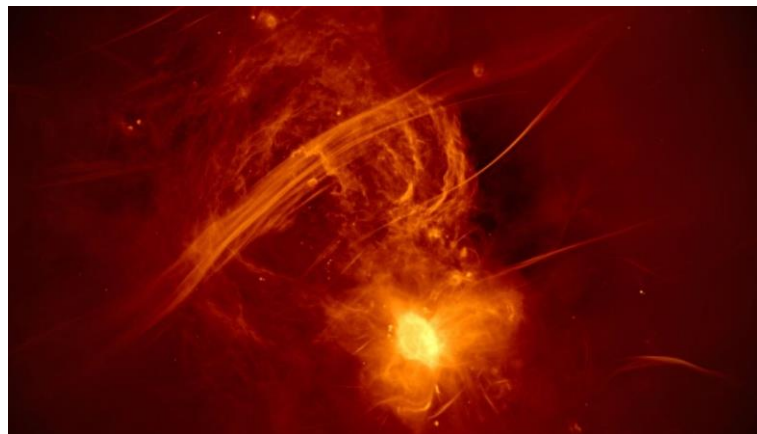
Рис.15. На зображенні показано перисте випромінювання від супербульбашики в центрі Чумацького Шляху, а найяскравіша точка – надмасивна чорна діра Стрілець А*.
