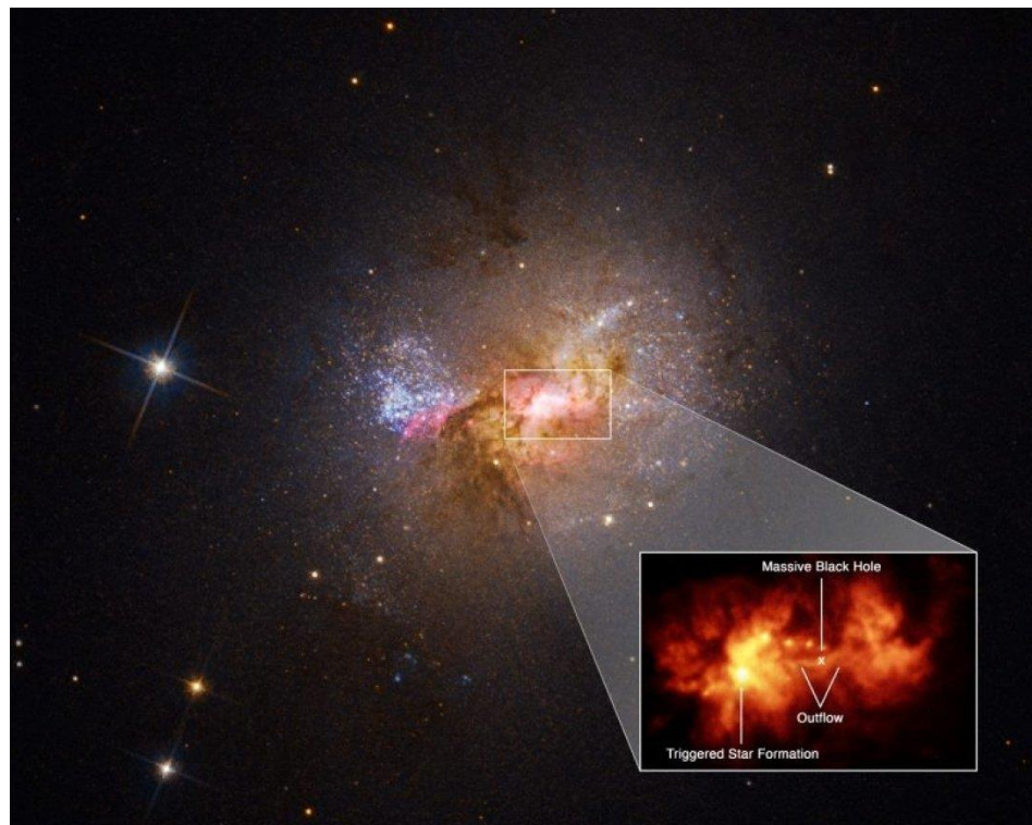
Рис.19. На зображенні центральної ділянки карликової галактики Henize 2-10 простежується потік гарячого газу довжиною 230 світлових років, що сполучає чорну дірку галактики та ділянку зіркоутворення
