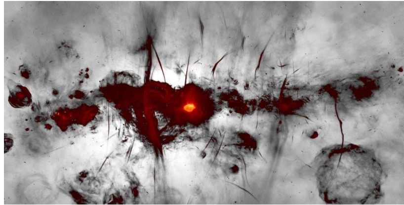
Рис.14. Виявлені структури мають величезні розміри та складаються з магнітних ниток, упорядкованих надзвичайно точно.
