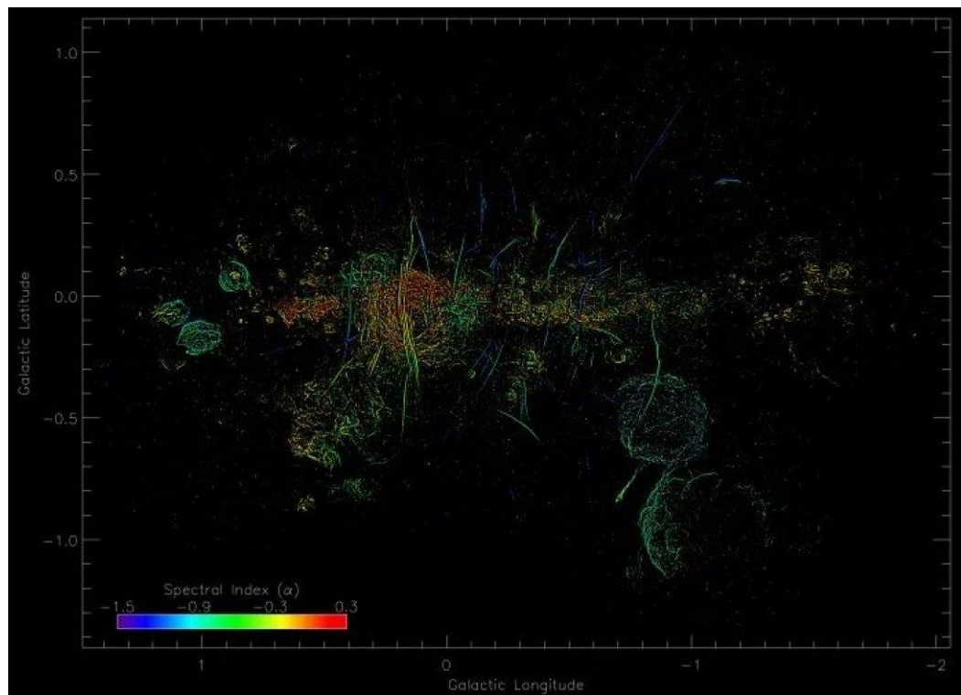
Рис.17. Карта магнітних ниток у галактичному центрі
