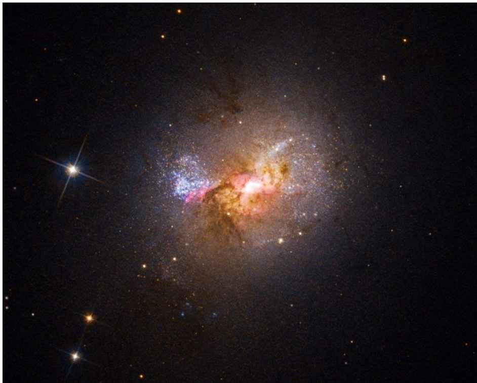
Рис.20. Карликова галактика Henize 2-10. Яскрава ділянка в центрі, оточена рожевими хмарами та темними смугами пилу, вказує на розташування чорної діри та ділянок зіркоутворення.
