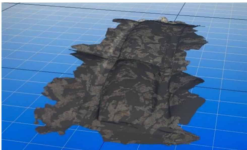
Рис.22. Вперше зроблена 3-д зйомка лідаром колій
