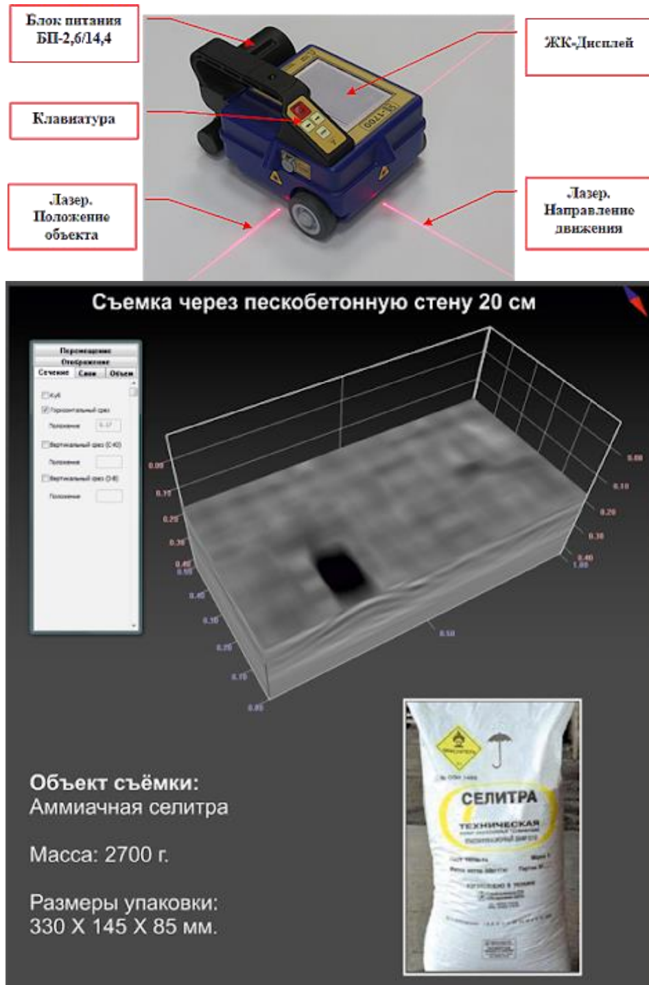
Рис.11. Вигляд і приклад локалізації прихованих об'єктів за допомогою георадару-бетоноскопу.
