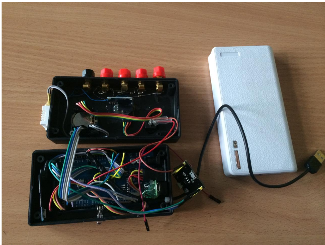
Рис.13. Прототип приладу
